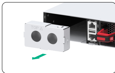
拆卸假面板
