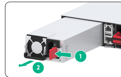
拆卸电源模块
